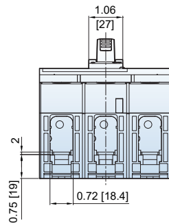
Bolt-on type
