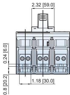
Bolt-on type
