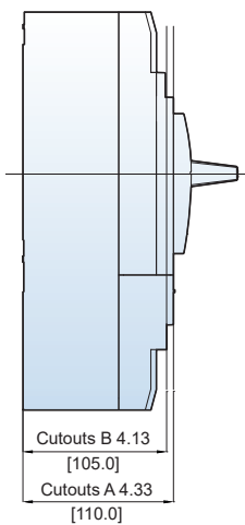
Door cutouts
