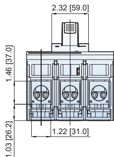
Lug type
