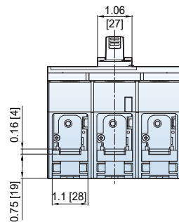
Bolt-on type
