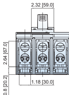
Lug type
