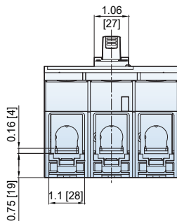
Lug type
