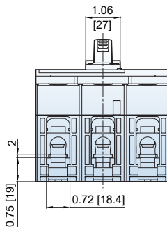
Lug type
